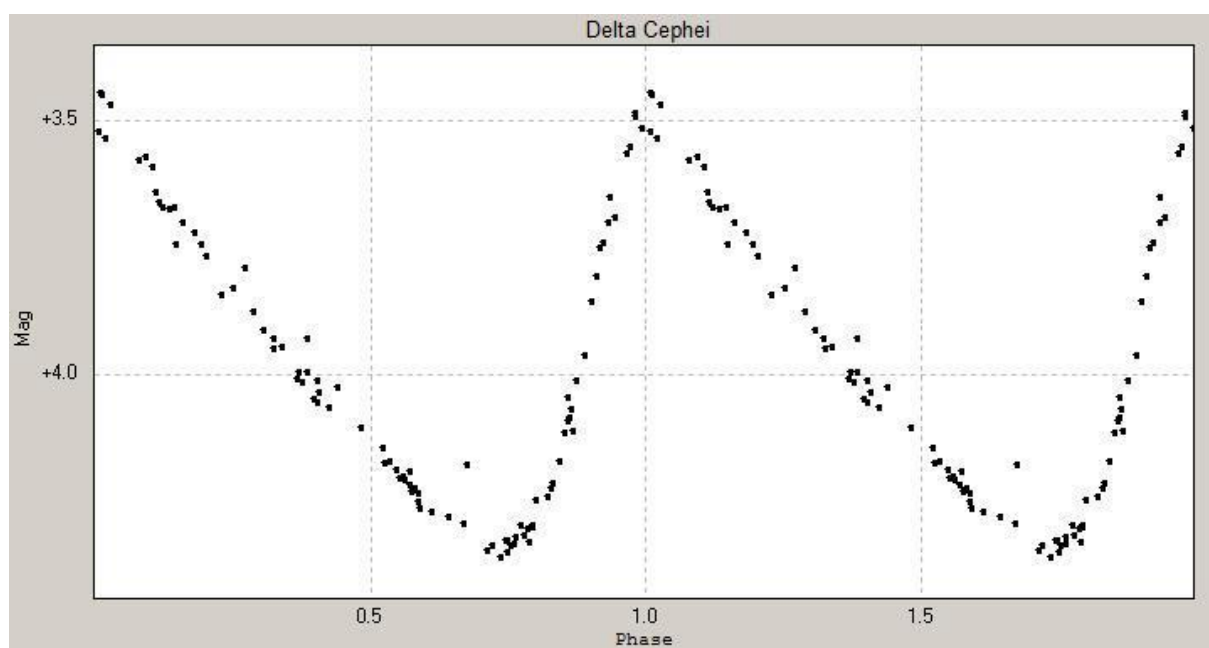
Фиг. 2. Крива на изменение на бляска на \delta Сер.
